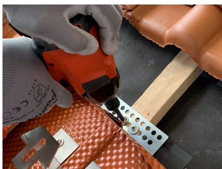
mit Sparrenschrauben befestigen
