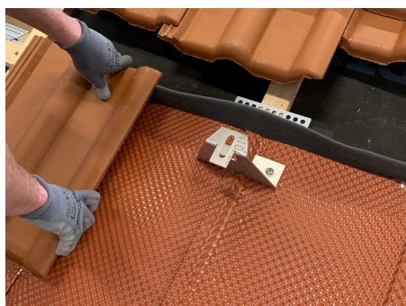
PV flex mit Haken einlegen
